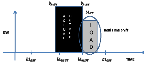
Fig A(5) Actual Load Schedule
